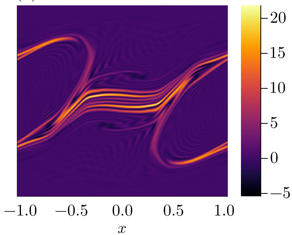
(d) \varepsilon = 10^{-10}
