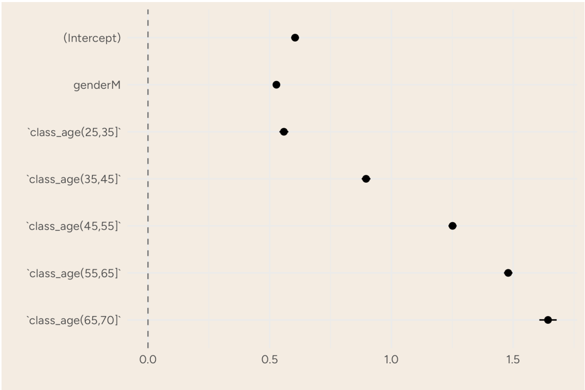
Figura 2.1: Grafico con i coefficienti del modello Quasi-Poisson
