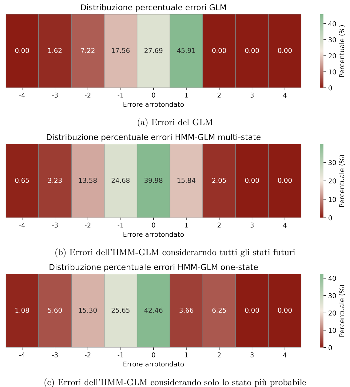
Figura 3.8: Mappe di calore sulla frequenza degli errori per i modelli testati
