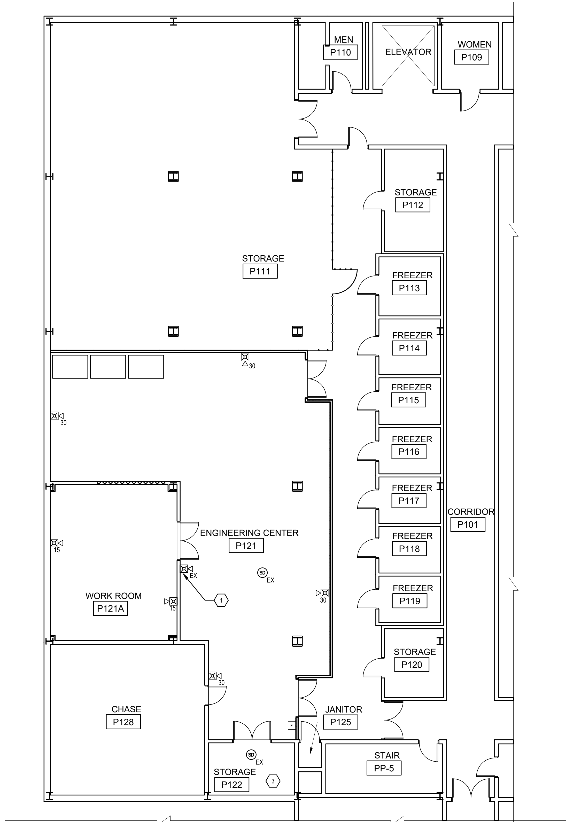
1 FIRE ALARM PLAN F-101 SCALE: 1/8"= 1'-0"
