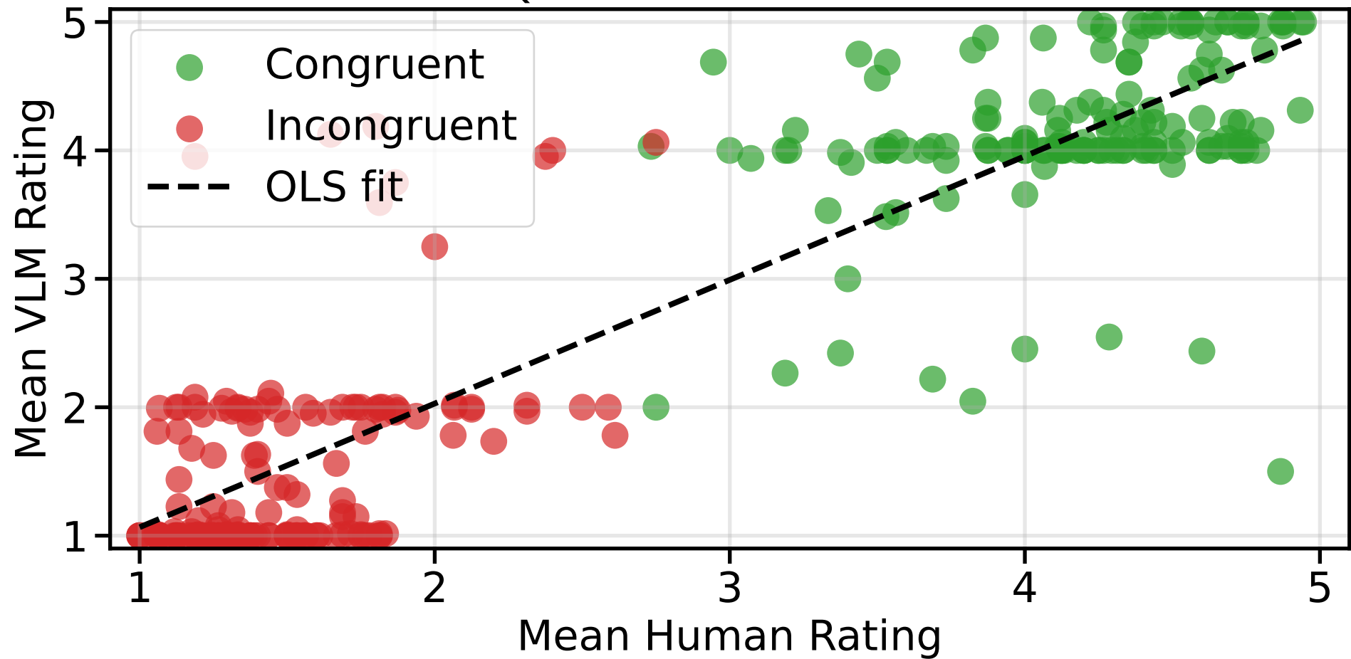
Qwen3-VL-4B-Instruct
