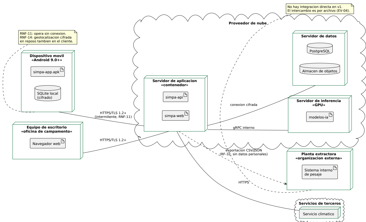
Figura 13: Diagrama de despliegue del SIMPA.
