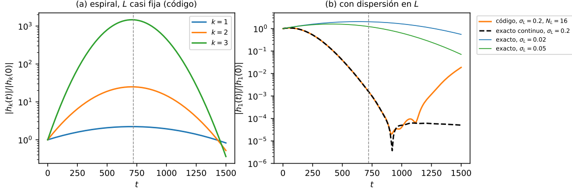
Figura 5: (a) Espiral con L casi fijo ( L \in [1.9995, 2.0005] ), código con analytic : los tres armónicos alcanzan su máximo en t = 710 (línea: t^* lineal). (b) Con dispersión en L . Negro discontinuo: exacto continuo con \sigma_L = 0.2 ; el desenrollado desaparece y |h_1| cae a 2.2 \times 10^{-3} en t = 700 . Naranja: el código con N_L = 16 , idéntico a la suma discreta, que se separa del continuo desde t \approx 1100 y sube: recurrencia por muestreo en L . Azul y verde: exacto continuo con \sigma_L = 0.02 y 0.05 .
