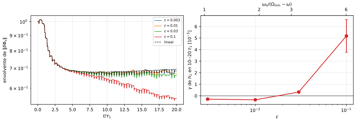
Figura 3: El barrido en \varepsilon del modo de L5. Izquierda: envolventes de \|\delta\Phi_\varepsilon\| a cuatro amplitudes y la teoría lineal. Derecha: \gamma de h_1 en 10\text{--}20\tau_1 frente a \varepsilon , con el cociente \omega_b/(\Omega_{\text{mín}} - \omega) arriba. Numérica: N = 400 \times 25 , \Delta t = 0.05 .
