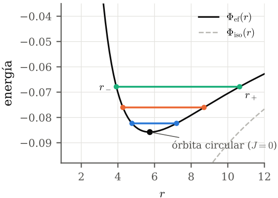
(a) potencial efectivo, L_0 = 2
