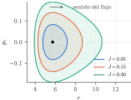
(b) órbitas: área encerrada = 2\pi J
