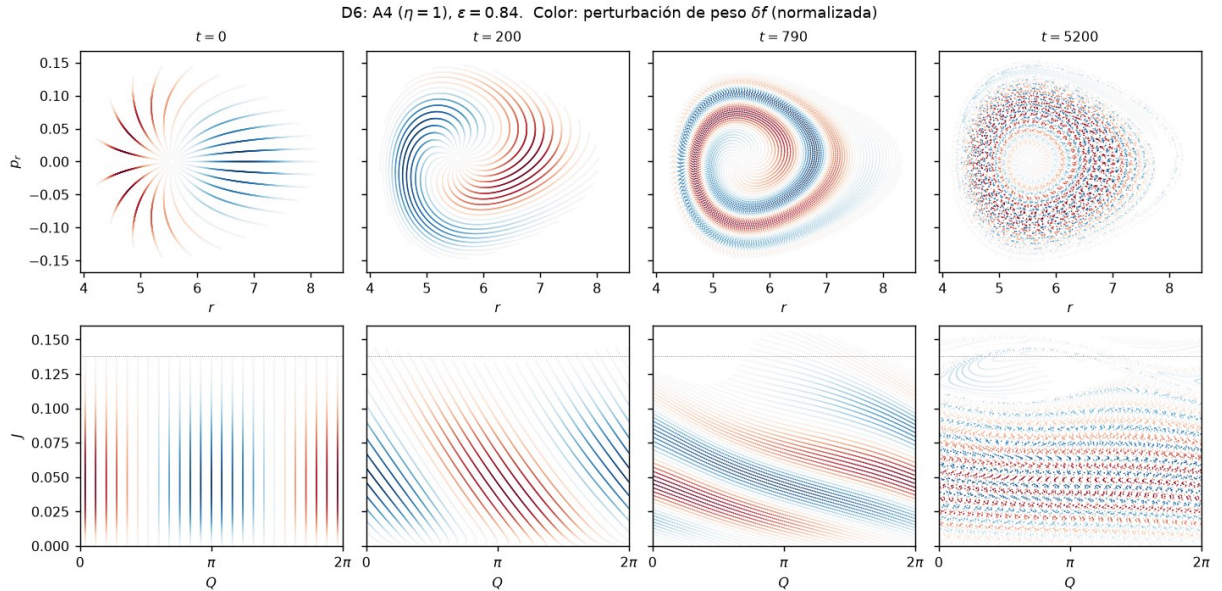
Figura 15: D6: \eta = 1 , \varepsilon = 0.84 . Al final ( t = 5200 ) las filas con J \gtrsim 0.11 se enrollan alrededor de un punto: la isla de partículas atrapadas por la onda, junto a la resonancia \Omega(J) = \omega cerca del borde. El cambio de acción llega a 0.048.
