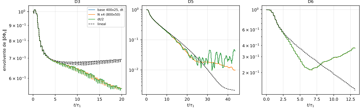
Figura 11: Convergencia de D3, D5 y D6: envolvente de \|\delta\Phi_\epsilon\| con la resolución de la demo ( 400 \times 25 , \Delta t = 0.05 ), con cuatro veces más partículas ( 800 \times 50 ) y con \Delta t/2 ; en trazos, la teoría lineal. La curva de \Delta t/2 tapa a la de la demo en los tres casos. En D5, la de N \times 4 se separa de las otras dos después de \sim 20\tau_1 .
