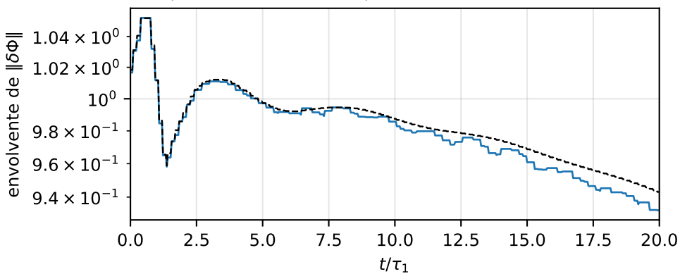
D4: \eta = 2 , modo discreto separado de la banda
