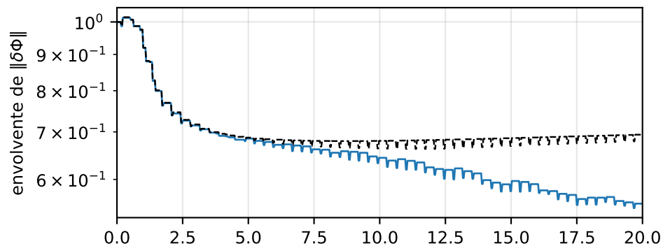
D4: \eta = 2 , modo discreto separado de la banda
