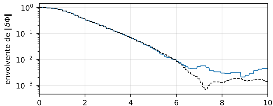
D3: \eta = 1.24 , modo discreto junto al borde, amplitud chica
