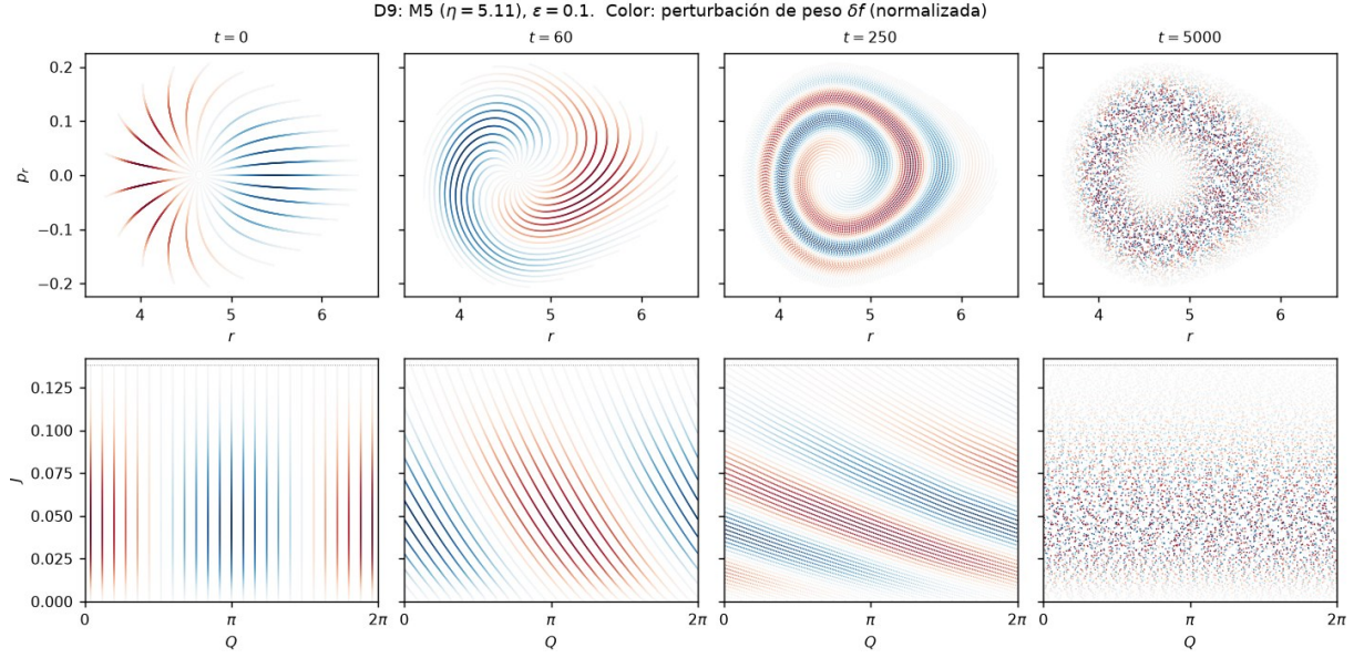
Figura 16: D9: a_0 = 0.5 ( \eta = 5.1 ), \varepsilon = 0.1 . La componente es más compacta ( r \in [3.6, 6.4] ) y las órbitas giran más rápido. Mezcla libre en las partículas, aunque el potencial sigue oscilando sin amortiguarse: las filas de J quedan horizontales (cambio máximo de acción 0.003).
