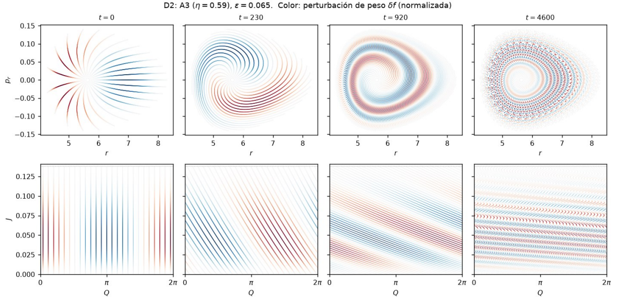
Figura 9: D2: \eta = 0.59 , \varepsilon = 0.065 . Igual que D1 con una perturbación quince veces menor; el modo colectivo se amortigua más despacio, pero en (Q, J) no se nota: la amplitud es chica.
