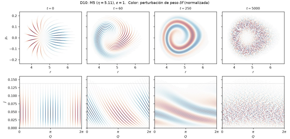
Figura 17: D10: a_0 = 0.5 , \varepsilon = 1 . Las filas se ondulan un poco en t = 250 y algunas partículas cruzan el borde J_t , hasta J = 0.157 , pero no se forma una isla: la resonancia del modo está en J \approx 0.22 .
