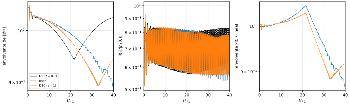
Figura 7: M5 ( a_0 = 0.5 , \eta = 5.1 ) a dos amplitudes: D9 ( \varepsilon = 0.1 ) y D10 ( \varepsilon = 1 ). El eje vertical de la izquierda abarca solo de 0.9 a 1.05: la envolvente se modula unos \pm 7\% por un batido lento que también tiene la teoría lineal. En la PIC el batido es más lento, y por eso el cociente de la derecha oscila; no hay amortiguamiento.
