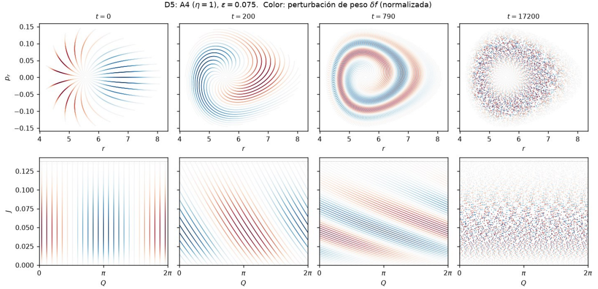
Figura 12: D5: \eta = 1 , \varepsilon = 0.075 , hasta t = 17200 ( 43 \tau_1 ). El cambio de acción se concentra junto al borde y se satura en 0.006: demasiado chico para verse a esta escala, pero unas quince veces el de la corrida sin perturbación.
