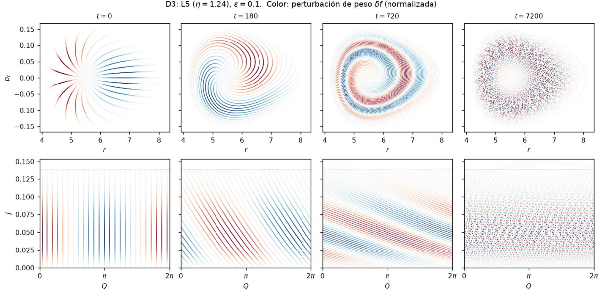
Figura 10: D3: \eta = 1.24 , \varepsilon = 0.1 , modo discreto pegado al borde. En (Q, J) las filas del borde ( J \approx 0.13 ) se despegan hacia afuera del soporte; su acción cambia hasta en 0.02 al final (ampliación en la figura 3).
