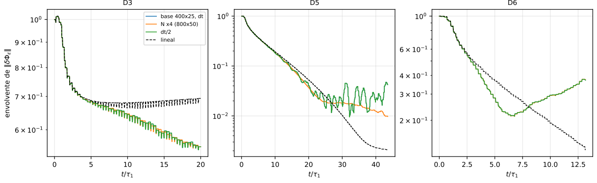
Figura 11: Convergencia de D3, D5 y D6: envolvente de \|\delta\Phi_\varepsilon\| con la resolución de la demo ( 400 \times 25 , \Delta t = 0.05 ), con cuatro veces más partículas ( 800 \times 50 ) y con \Delta t/2 ; en trazos, la teoría lineal. La curva de \Delta t/2 tapa a la de la demo en los tres casos. En D5, la de N \times 4 se separa de las otras dos después de \sim 20 \tau_1 .
