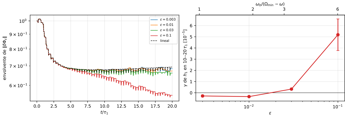
Figura 3: El barrido en \varepsilon del modo de L5. Izquierda: envolventes de \|\delta\Phi_\varepsilon\| a cuatro amplitudes y la teoría lineal. Derecha: \gamma de h_1 en 10 – 20\tau_1 frente a \varepsilon , con el cociente \omega_b/(\Omega_{\min} - \omega) arriba. Numérica: N = 400 \times 25 , \Delta t = 0.05 .
