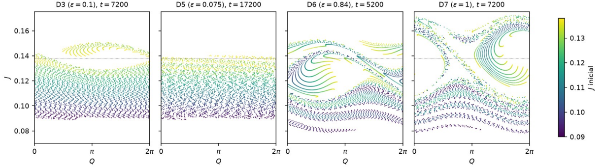
Figura 4: El borde de la banda al final de cuatro corridas: las partículas con J_0 > 0.09 en (Q, J) , coloreadas por su acción inicial . En la mezcla libre cada color quedaría en su fila horizontal; la línea punteada es el borde del soporte, J_t . D3: las filas del borde se despegan y forman un arco fuera del soporte, hasta J = 0.151 . D5: el cambio es chico ( J \leq 0.140 ). D6 y D7: islas de partículas atrapadas, con su punto X y curvas cerradas alrededor del centro, que se extienden hasta J = 0.153 y 0.179 . La posición de la isla en Q gira con la onda y no tiene significado.
