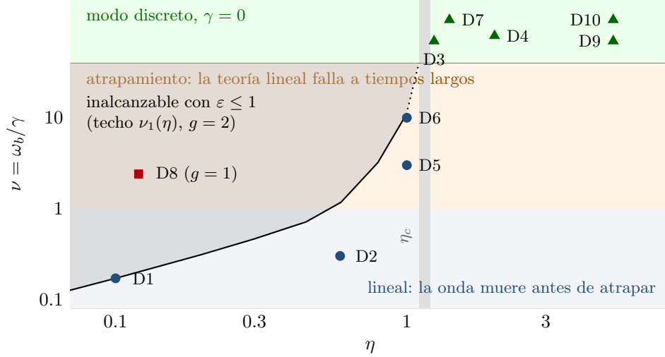
Figura 1: Las corridas en el plano (\eta, \nu) . La franja gris es la transición lineal, \eta_c \approx 1.1 – 1.2 . La curva negra es el techo \nu_1(\eta) = \omega_b(\varepsilon = 1)/\gamma de la familia con g = 2 (tabla 2; punteada, la extrapolación hacia \eta_c , donde \gamma \rightarrow 0 ): con esta perturbación no se puede estar por encima, y la zona sombreada es inalcanzable (sección 2.2). D1 está sobre el techo ( \varepsilon = 1 ). D8 es de otra familia ( g = 1 ), con un techo propio más alto porque su decaimiento tardío es lento. Arriba, fuera de escala, los modos discretos: ahí no hay partículas resonantes y \nu no aplica (D3 y D7 están en el mismo \eta , separadas para que se lean; lo mismo D9 y D10). D8 está desplazada un poco en \eta respecto de D1. El eje de \eta es logarítmico.
