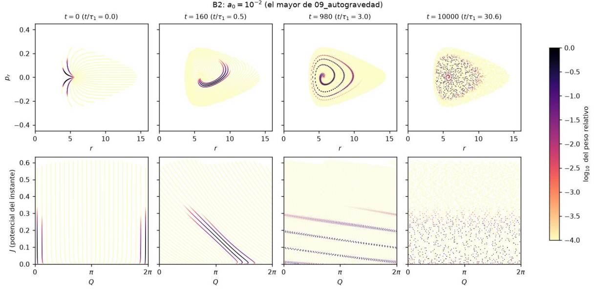
Figura 19: B2: el bulto con a_0 = 10^{-2} , la masa mayor de las corridas originales. Color: logaritmo del peso de cada partícula (oscuro, donde está la masa). Se cizalla en espiral y se mezcla, pero al final queda un resto de núcleo en r \approx 5.7 . Abajo, (Q, J) en el potencial de cada instante.
