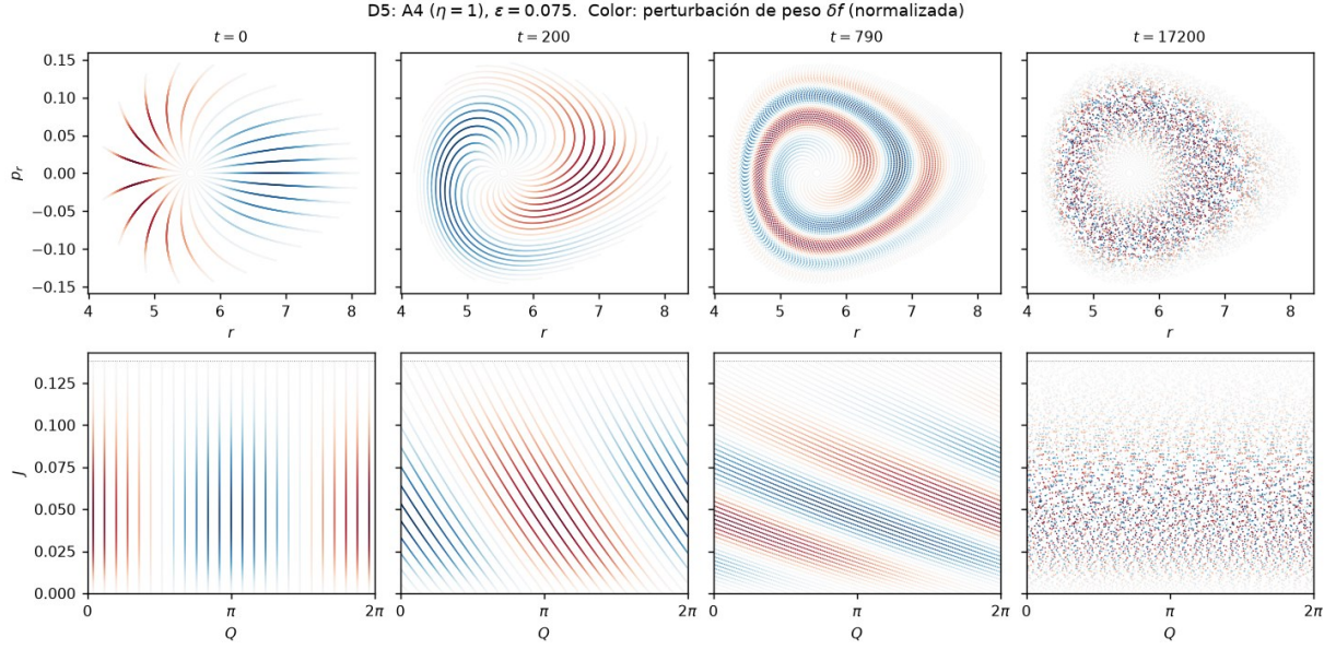
Figura 13: D5: \eta = 1 , \varepsilon = 0.075 , hasta t = 17200 ( 43 \tau_1 ). El cambio de acción se concentra junto al borde y se satura en 0.006: demasiado chico para verse a esta escala, pero unas quince veces el de la corrida sin perturbación.
