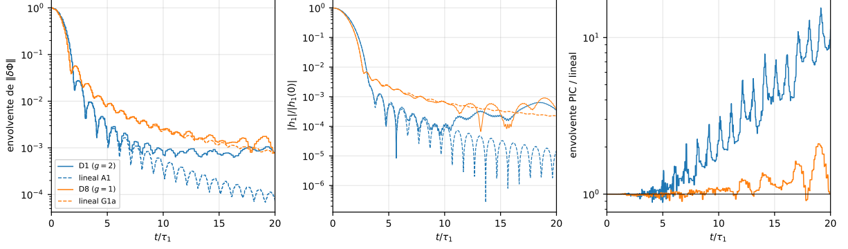
Figura 4: El mismo \eta = 0.1 con borde suave (D1, g = 2 ) y abrupto (D8, g = 1 ). Izquierda y centro: envolvente de \|\delta\Phi\| y |h_1| ; en trazos, la teoría lineal de cada equilibrio. Derecha: cociente de envolventes PIC/lineal. D1 llega al piso de la medida hacia 5\tau_1 (§3.6); D8 queda por encima hasta \sim 15\tau_1 .
