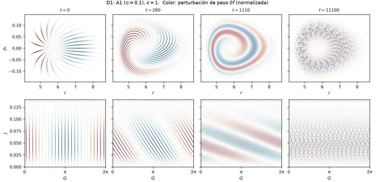
Figura 9: D1: \eta = 0.1 , \varepsilon = 1 . La mezcla libre casi pura: las filas de J siguen horizontales; el cambio máximo de acción es 0.002.
