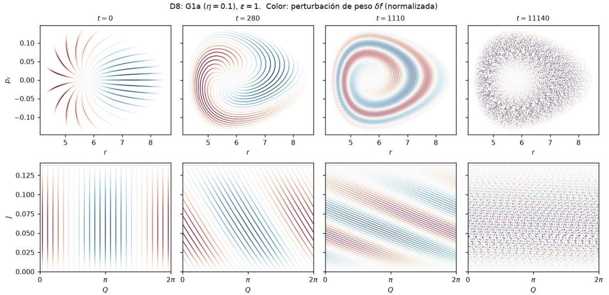
Figura 16: D8: \eta = 0.1 , \varepsilon = 1 , borde abrupto ( g = 1 ). Como D1: en espacio fase la diferencia entre los bordes no se ve, porque la respuesta que persiste en el borde es de 10^{-3} del valor inicial.
