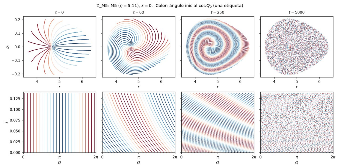
Figura 23: Referencia de M5 (D9 y D10).
