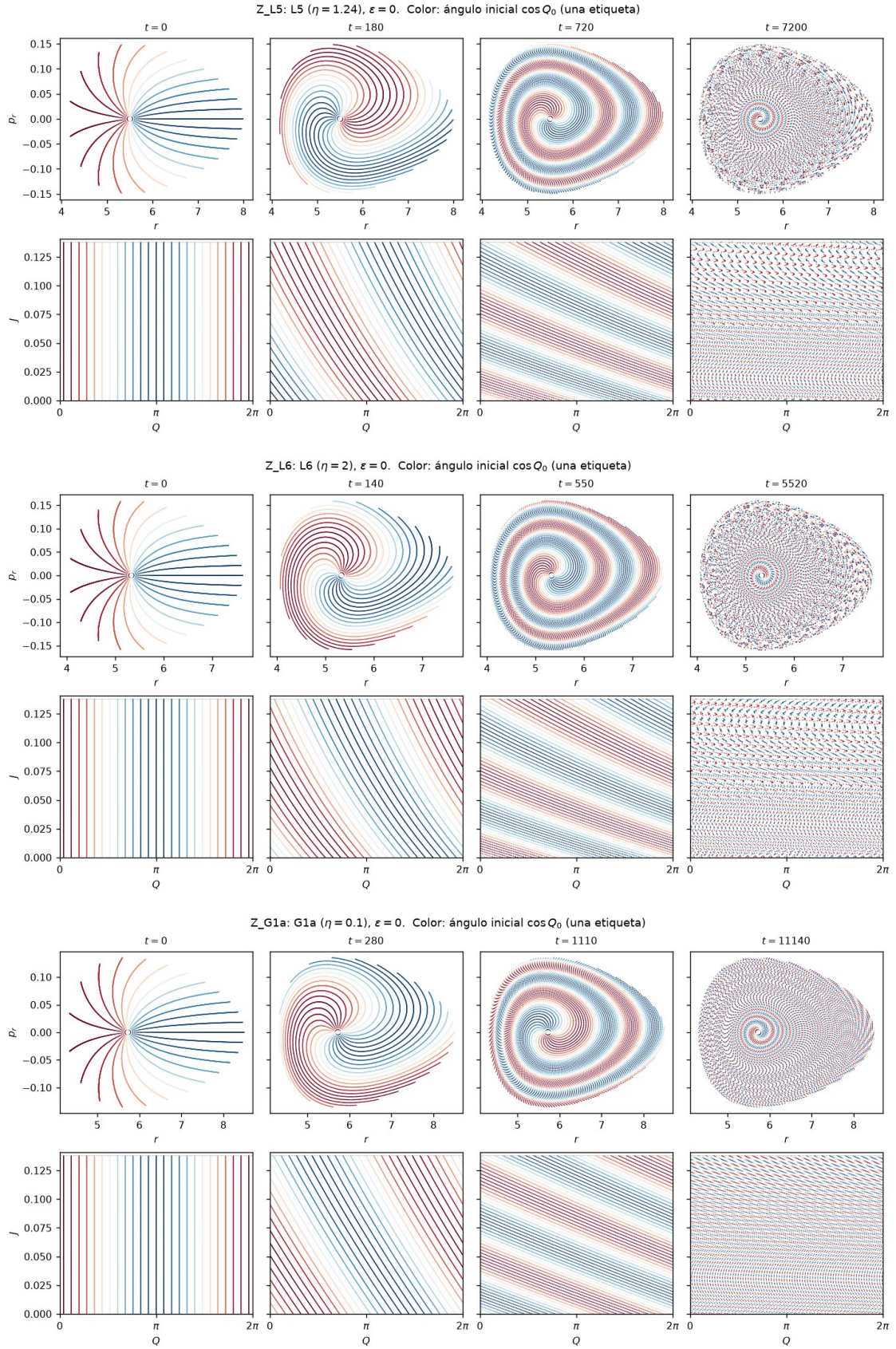
Figura 22: Referencias de L5 (D3 y D7), L6 (D4) y G1a (D8).
