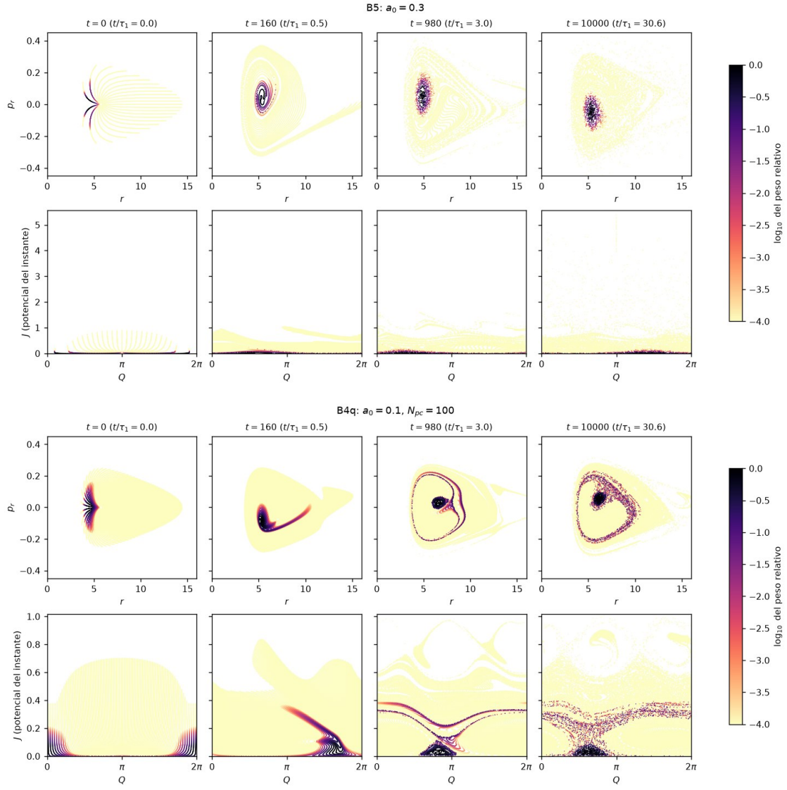
Figura 25: El bulto con a_0 = 0.3 (B5) y con a_0 = 0.1 y N_{pc} = 100 (B4q).
