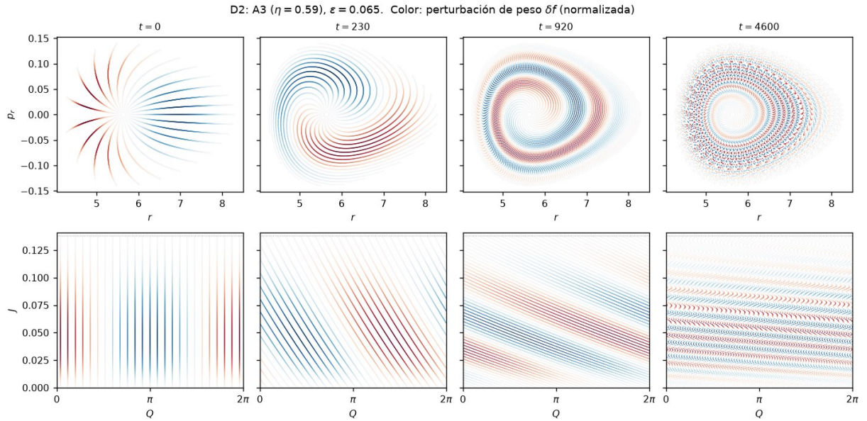
Figura 10: D2: \eta = 0.59 , \varepsilon = 0.065 . Igual que D1 con una perturbación quince veces menor; el modo colectivo se amortigua más despacio, pero en (Q, J) no se nota: la amplitud es chica.
