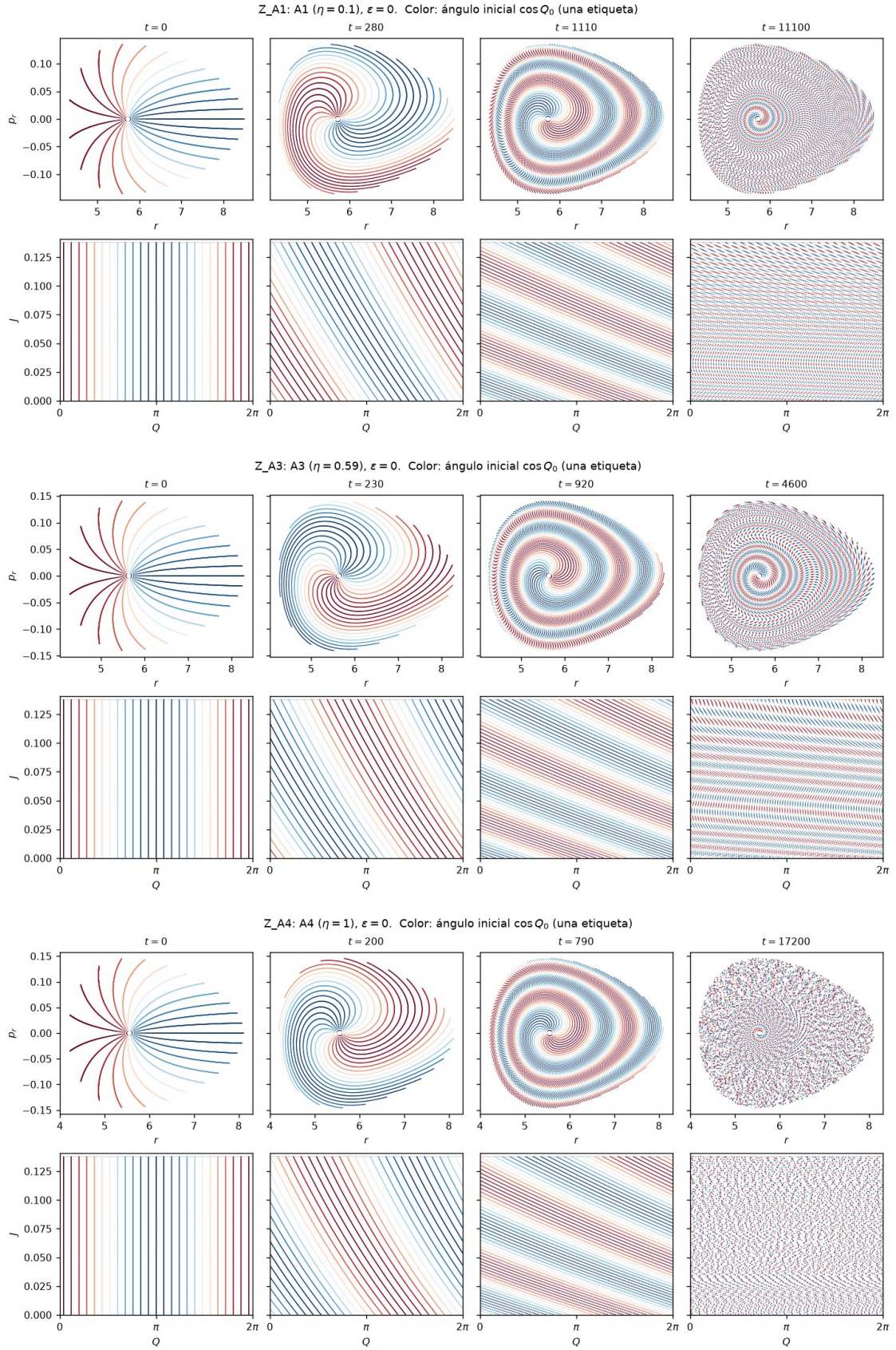
Figura 21: Referencias de A1 (D1), A3 (D2) y A4 (D5 y D6).
