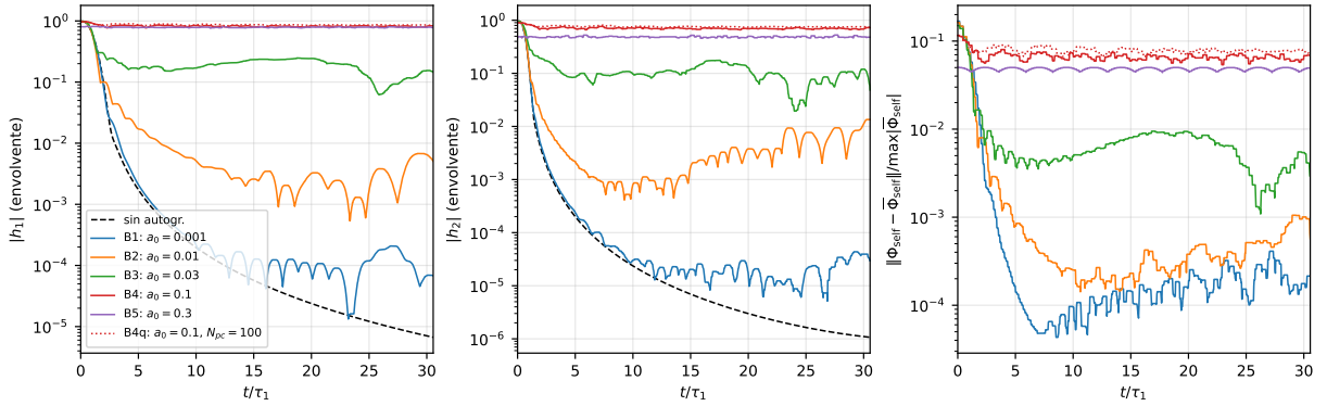
Figura 8: El bulto a distintas masas. Izquierda y centro: envolventes de |h_1| y |h_2| en el mapa del potencial del instante; en trazos, sin autogravedad. Derecha: fluctuación del potencial propio alrededor de su media tardía. Entre a_0 = 10^{-2} y 0.1 el comportamiento cambia de mezcla a bulto que no se deshace.
