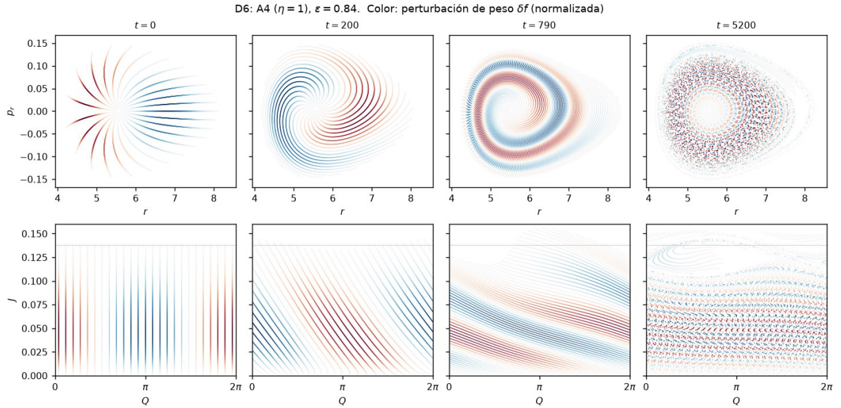
Figura 14: D6: \eta = 1 , \varepsilon = 0.84 . Al final ( t = 5200 ) las filas con J \gtrsim 0.11 se enrollan alrededor de un punto: la isla de partículas atrapadas por la onda, junto a la resonancia \Omega(J) = \omega cerca del borde. El cambio de acción llega a 0.048.
