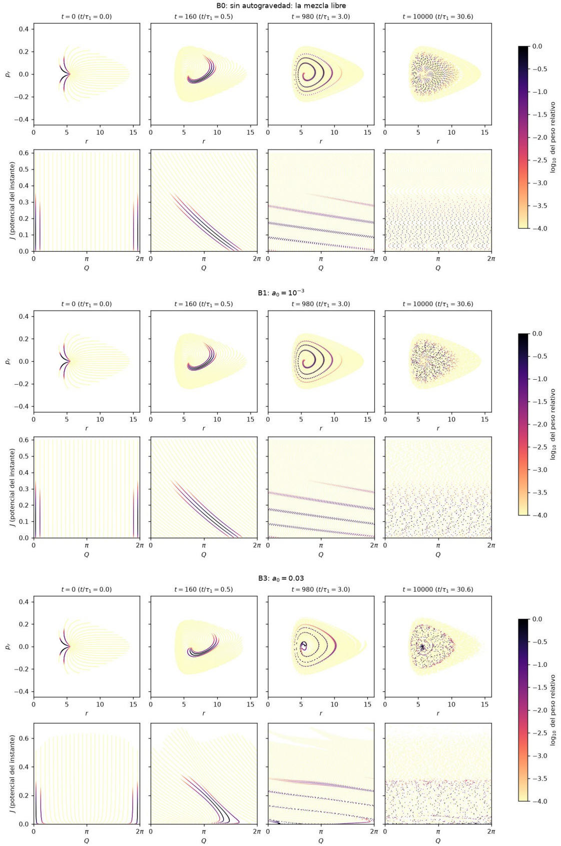
Figura 24: El bulto sin autogravedad (B0), con a_0 = 10^{-3} (B1) y con a_0 = 0.03 (B3).
