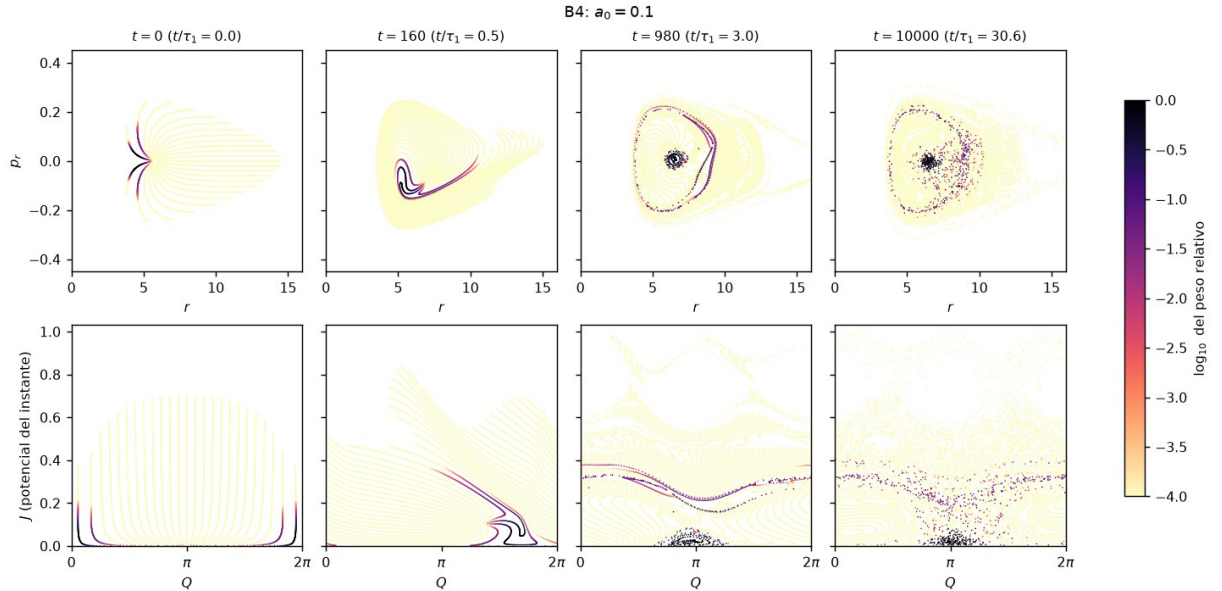
Figura 20: B4: el bulto con a_0 = 0.1 . Colapsa en las primeras vueltas en un núcleo denso ( r \approx 6.5 , p_r \approx 0 en estos instantes) con el 79 % de la masa, rodeado de un halo de partículas arrancadas. En (Q, J) el núcleo está en J \approx 0 : es la órbita casi circular del potencial que él mismo crea.
