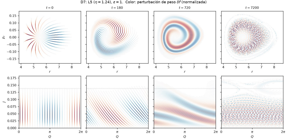
Figura 15: D7: \eta = 1.24 , \varepsilon = 1 . Ya en t = 720 las filas se ondulan, y al final hay una isla junto al borde, con partículas hasta J = 0.179 , fuera del soporte. El cambio de acción llega a 0.073, más de la mitad del soporte.
