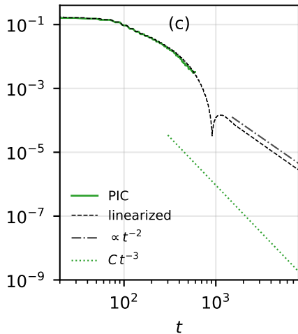
polytrope, k = 2 , M_{gas}/M = 1
