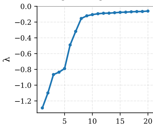
Negative eigenvalues
