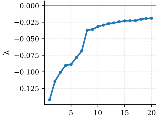
Negative eigenvalues
