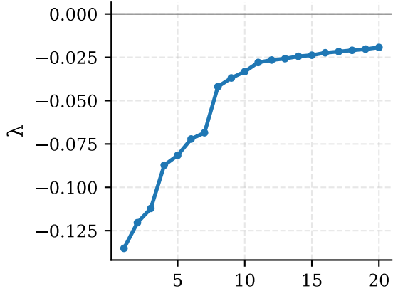
Negative eigenvalues
