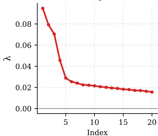
Positive eigenvalues
