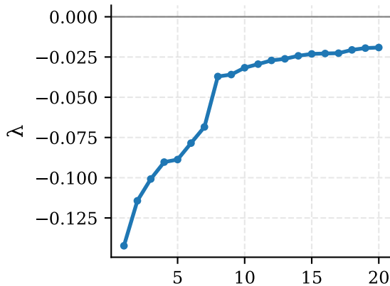
Negative eigenvalues
