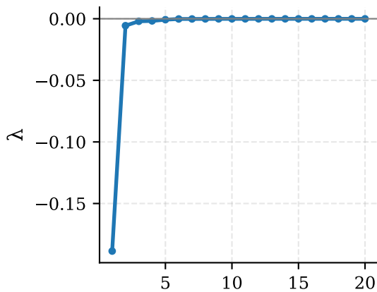
Negative eigenvalues
