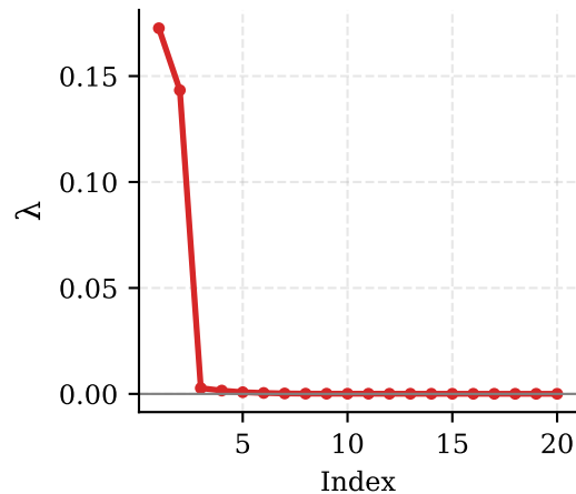
Positive eigenvalues
