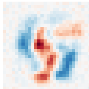
Class 2 (-2.39)
