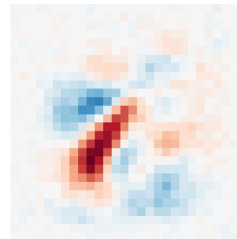
Class 9 (-3.76)
