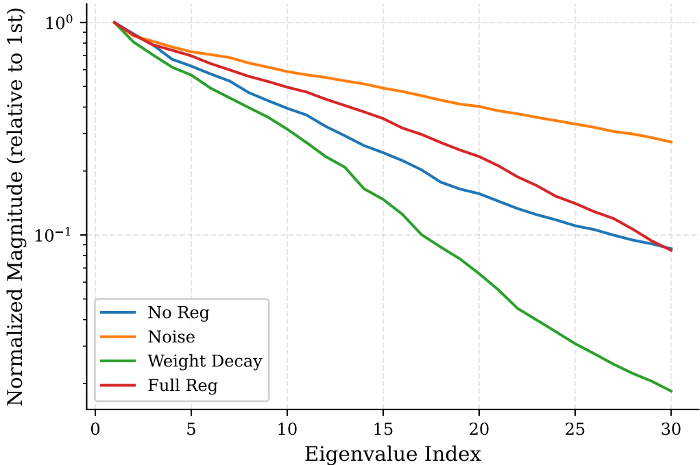
MNIST: Normalized Eigenvalue Decay
