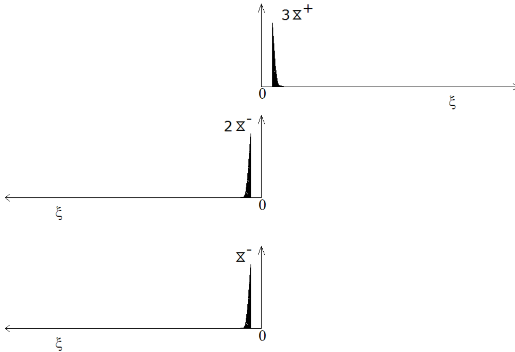
Figura 5.3. Número de épísimas par, pero no divisible por 4
