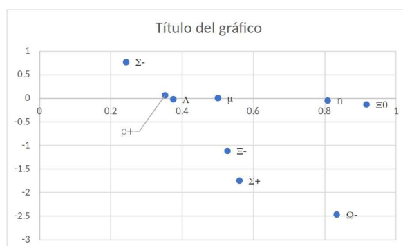
Figura 5.24. % error másico vs proporción de epísimas pesadas
