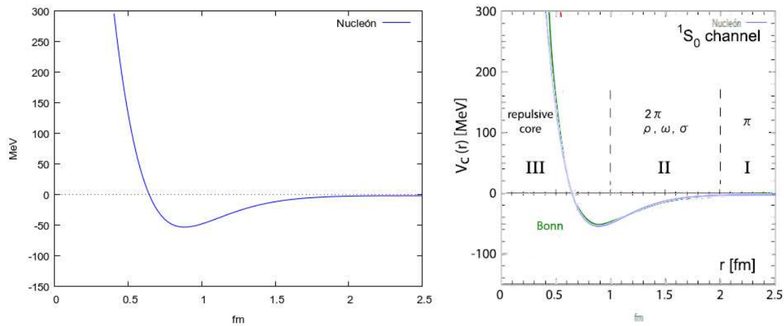
Figura 6.40. Media del potencial electrofuerte sin deformar y deformado. Superposición con datos experimentales
