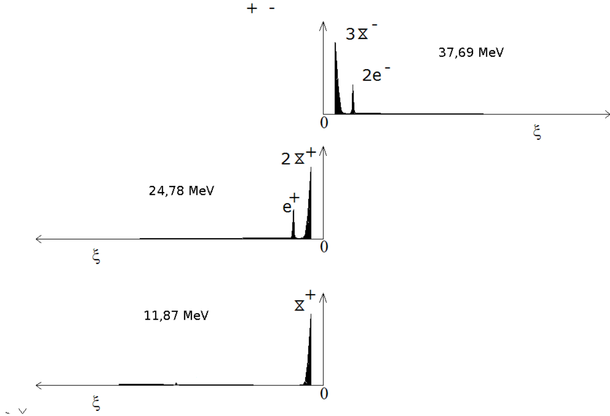
Figura 5.4. Propuesta para el muón
