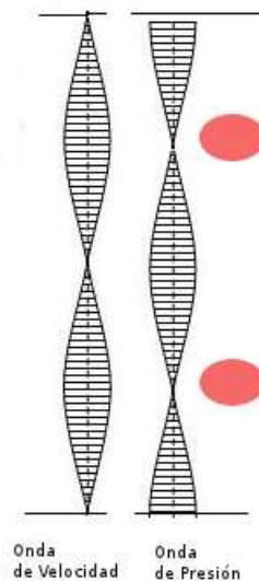
Figura 2.17. Levitación acústica
