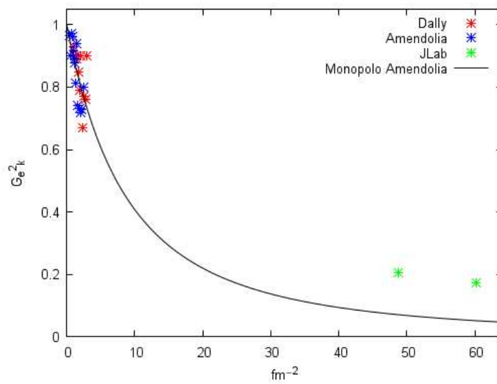
Figura 6.33. Factor de forma a bajo q^2
