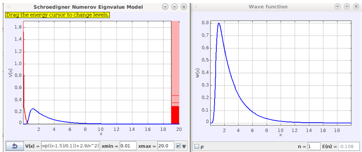
Figura 7.9. Función de onda del deuterón
