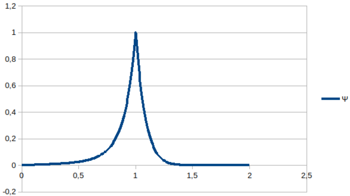
Figura 2.6. Solución cualitativa tipo III para q=-20
