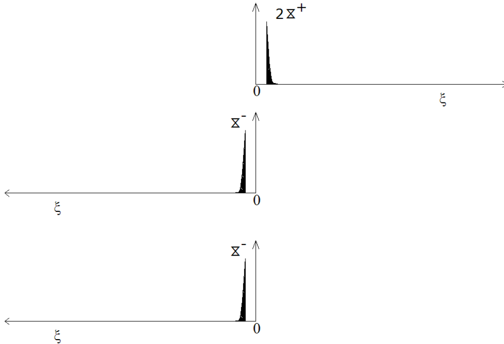
Figura 5.2. Tipo Helio. N° epísimas divisible por 4
