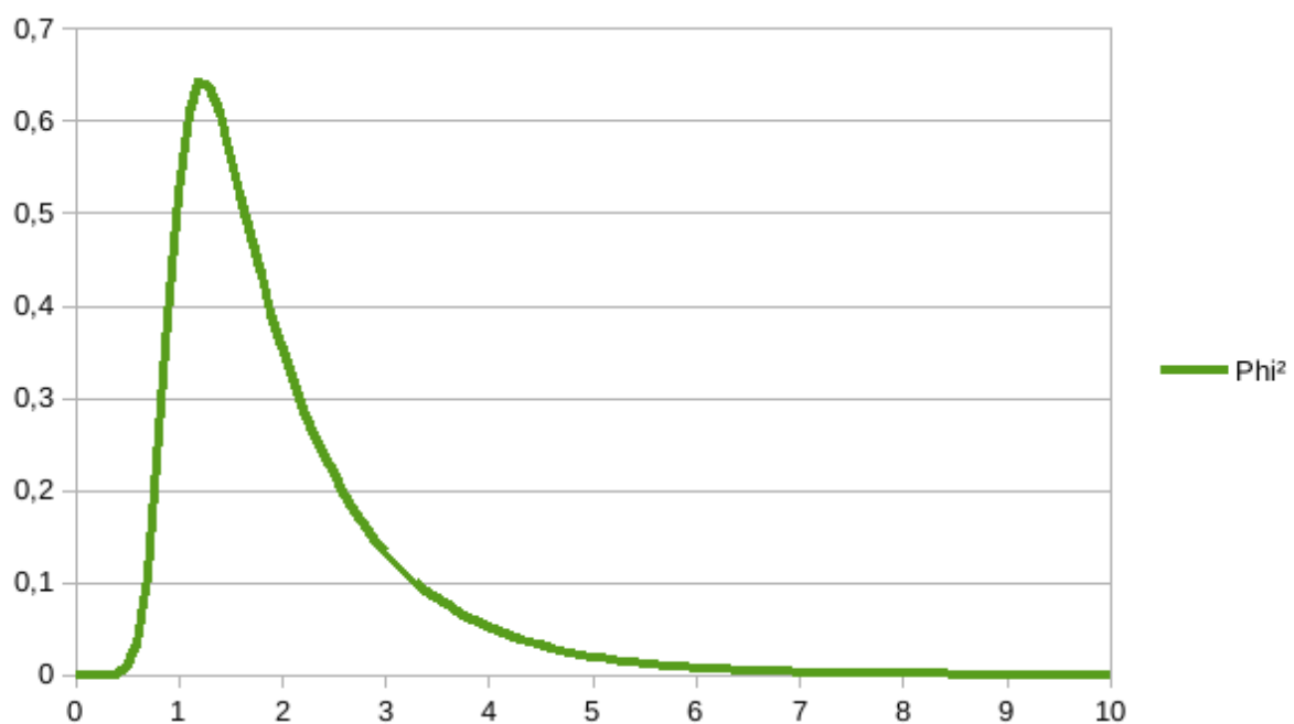
Figura 7.10. Función de onda estimada del deuterón
