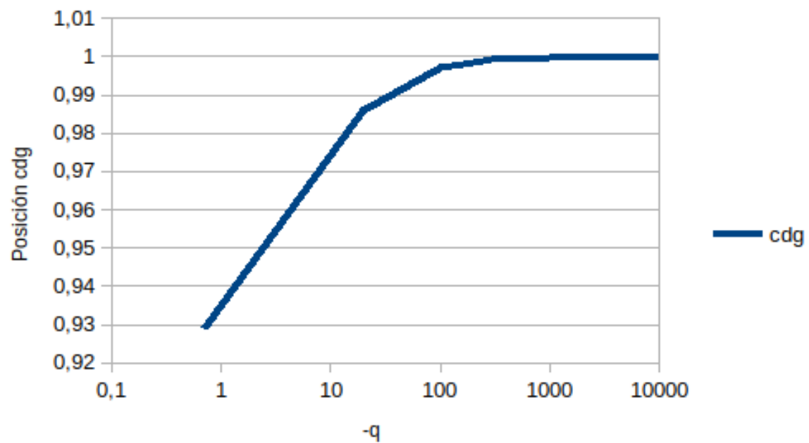
Figura 2.5. Solución tipo III. Posición del cdg
