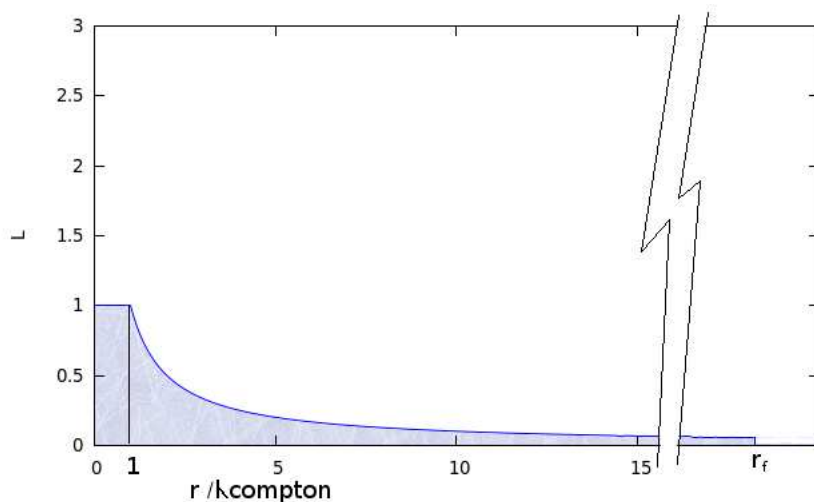
Figura 2.9. Solución en función de r para una partícula-pulsación inmóvil.
