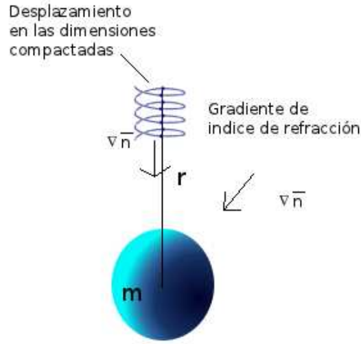
Figura 2.16. Origen de la curvatura del tiempo
