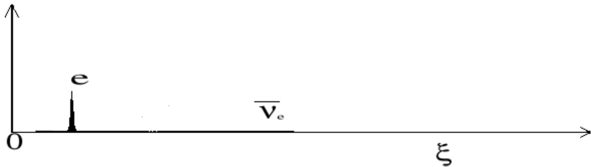
Figura 2.6. Las combinaciones lineales de las soluciones tipo III conformarían al electrón.
