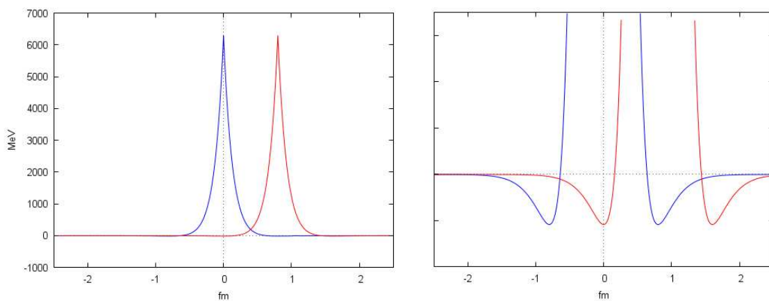
Figura 7.2. Dos protones a = 0,8 fm
