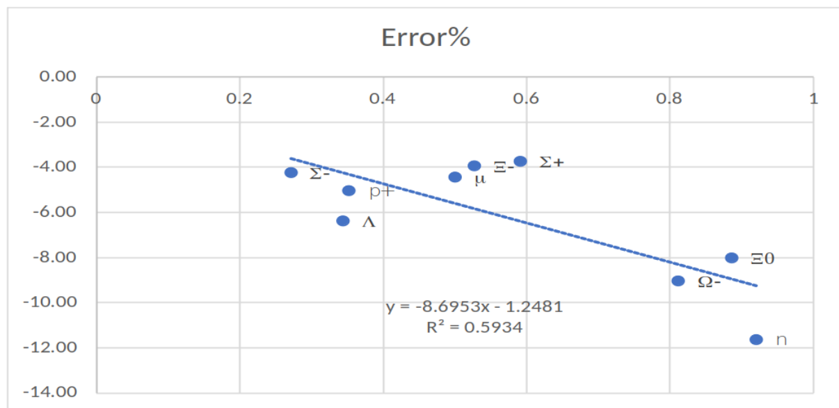
Figura 5.27. % error m. magnético vs proporción de epísimas pesadas
