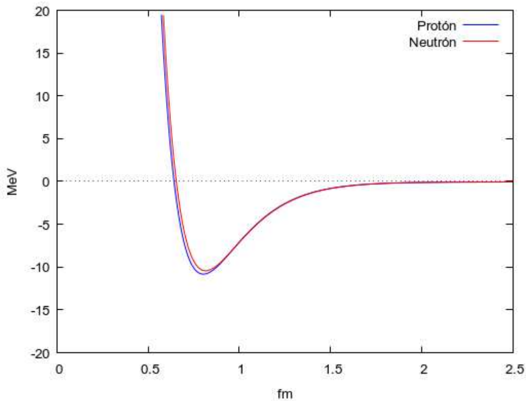
Figura 7.1. Potencial electrofuerte
