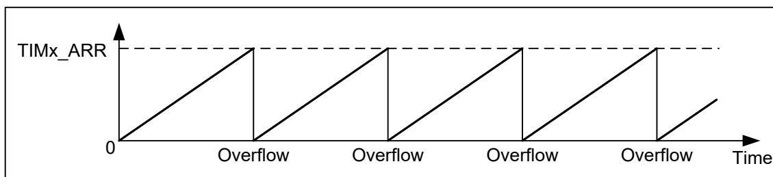
图 1-3 向上计数器
