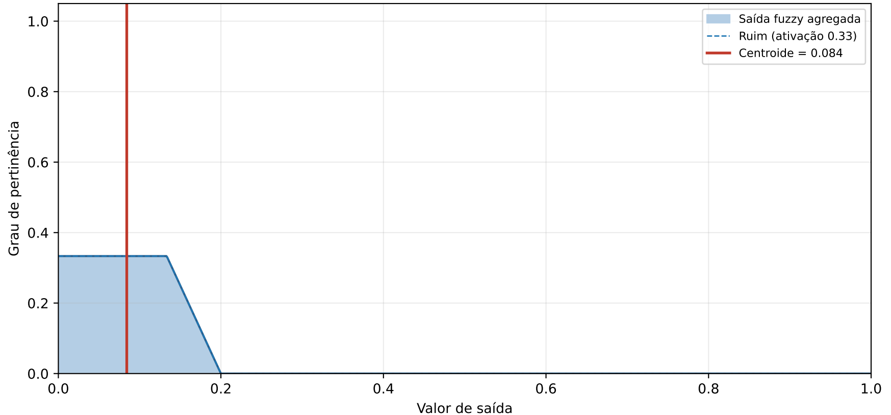
Conjunto fuzzy de saída e defuzzificação
