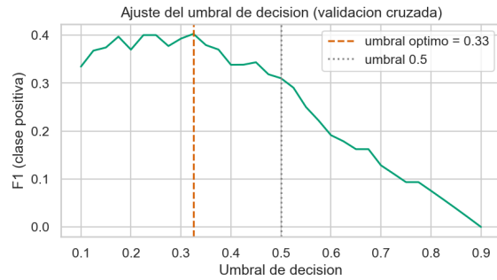
Figura 3. F1 de la clase positiva en función del umbral de decisión (validación cruzada). El óptimo (0.33) mejora claramente respecto al umbral por defecto 0.5.
