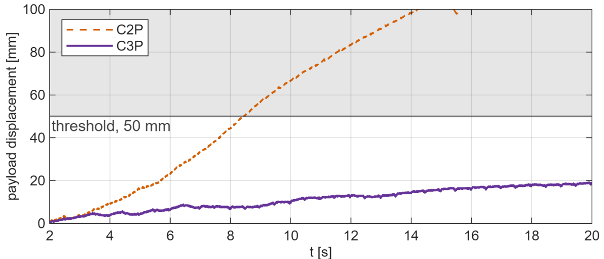
Figura 8: Spostamento del pacco dal riferimento sulla rampa di 8° (T4), con l’anello d’assetto spento (C2P) e acceso (C3P). La linea e la fascia grigia segnano il gioco di 50 mm fra cubo e vassoio: sopra, il cubo non è più contenuto dal vassoio. C2P lo supera dopo 8.4 s e prosegue senza tornare indietro — oltre il riquadro la curva arriva a decine di metri, perché il cubo lascia il robot e cade. C3P resta sotto i 20 mm per tutta la corsa. La misura parte da 2 s, dopo il transitorio di assestamento su cui è definito il riferimento.
