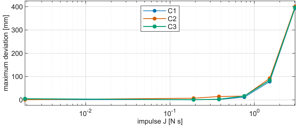
Figura 6: Deviazione laterale massima contro l’ampiezza dell’impulso applicato (T7), in scala logaritmica sull’ascissa per coprire le tre decadi della spazzata. Le tre curve sono praticamente indistinguibili su tutto l’intervallo: fino a circa 0.7 N s la deviazione resta di pochi millimetri per tutti, oltre cresce bruscamente fino a quasi 400 mm senza che nessuno dei tre controllori si distingua dagli altri. È la rappresentazione diretta di una lacuna architetturale comune: né la ricerca del terreno né l’anello d’assetto intervengono su questo disturbo.
