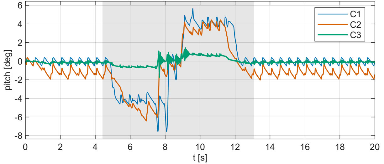
Figura 4: Beccheggio del corpo durante il superamento dell’ostacolo singolo (T5). In grigio la finestra in cui almeno un piede si trova sull’ostacolo, identificata cinematicamente. Fuori da quella finestra le tre curve oscillano attorno allo zero con l’ampiezza del passo; dentro, C1 e C2 compiono un’escursione di diversi gradi in entrambi i versi — prima il muso in su mentre le zampe anteriori salgono sul gradino, poi in giù quando vi salgono le posteriori — mentre C3 resta entro circa un grado per tutto il passaggio. È la stessa differenza che la Tabella 8 riporta come -73\% di beccheggio di picco.
