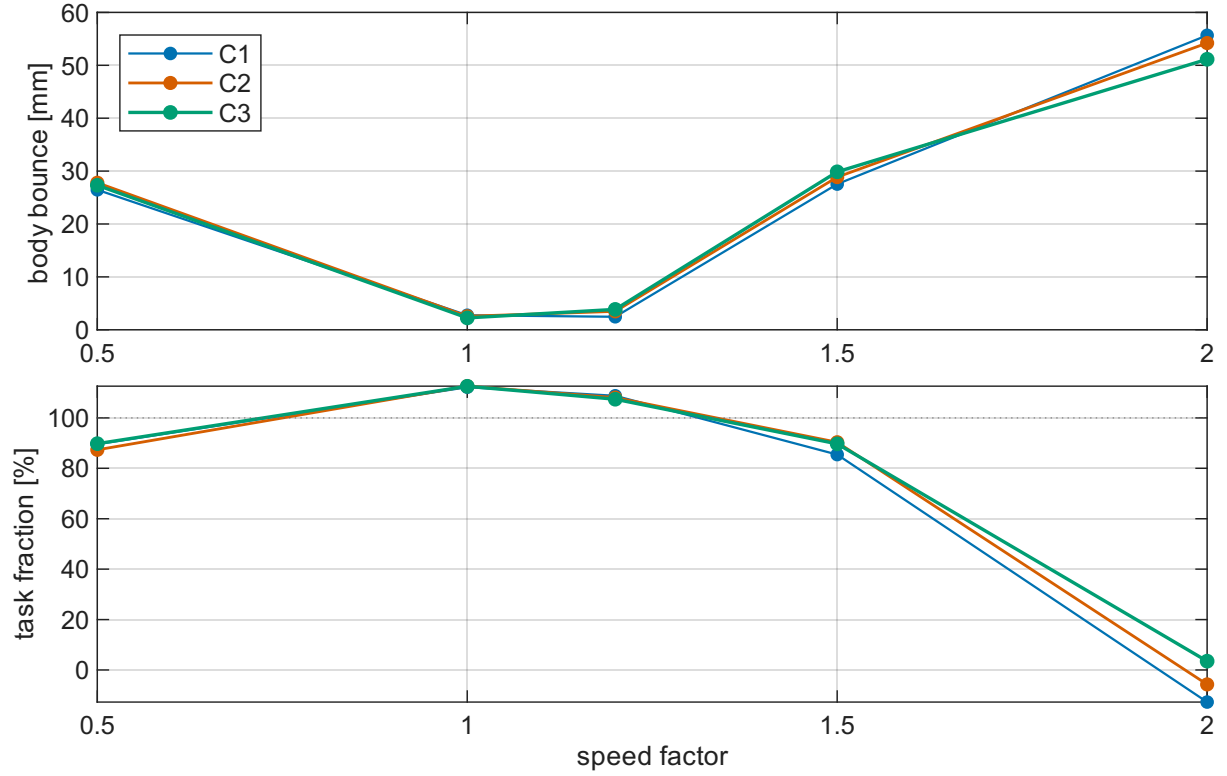
Figura 2: Spazzata in velocità (T2) per i tre controllori: rimbalzo verticale del corpo (sopra) e frazione del task percorsa (sotto) contro il fattore di velocità comandato.
