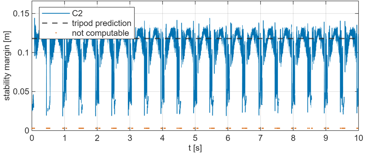
Figura 10: Margine di stabilità del controllore C2 in marcia rettilinea in piano (T2) a velocità nominale (0.12 m/s, periodo 1 s), per dieci cicli. Il margine è la distanza con segno dello ZMP dal lato più vicino del poligono formato dai piedi d'appoggio: positivo se lo ZMP è interno al poligono.
