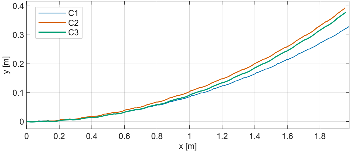
Figura 3: Traiettorie del centro di massa nel piano orizzontale con comando di imbardata +0.1 \text{ rad/s} (T3). Le tre curve si sovrappongono quasi ovunque: il comando di imbardata viene seguito allo stesso modo dai tre controllori, e le differenze della Tabella 7 su questo task riguardano l’assetto del corpo, non il percorso. Le scale dei due assi sono diverse — quasi due metri in ascissa contro quattro decimetri in ordinata — quindi lo scostamento laterale appare molto più marcato di quanto sia.
