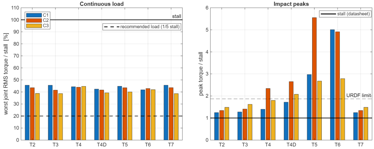
Figura 7: Coppia richiesta ai giunti contro i limiti dell’AX-12A, per task e controllore. Vanno letti due regimi distinti: la coppia efficace del giunto più caricato, che descrive la marcia e resta stabilmente sotto lo stallo ma sopra il carico continuo raccomandato dal costruttore, e la coppia di picco, che lo stallo lo supera in corrispondenza degli urti all’appoggio. I valori numerici corrispondenti sono nella Tabella 12.
