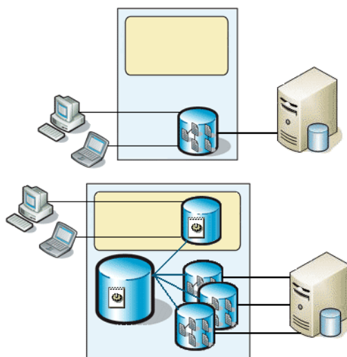
Figura 3. Sitio de un solo nodo con un servidor de aplicaciones, y otro sitio con dispatcher y controller y varios servidores de aplicaciones.
