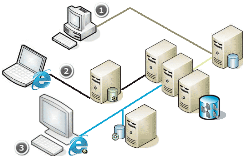
Figura 2. Representación de la arquitectura de Cegid. Se incluyen los clientes Windows (1), los clientes HTML (2) y los clientes Rich Web (3).
