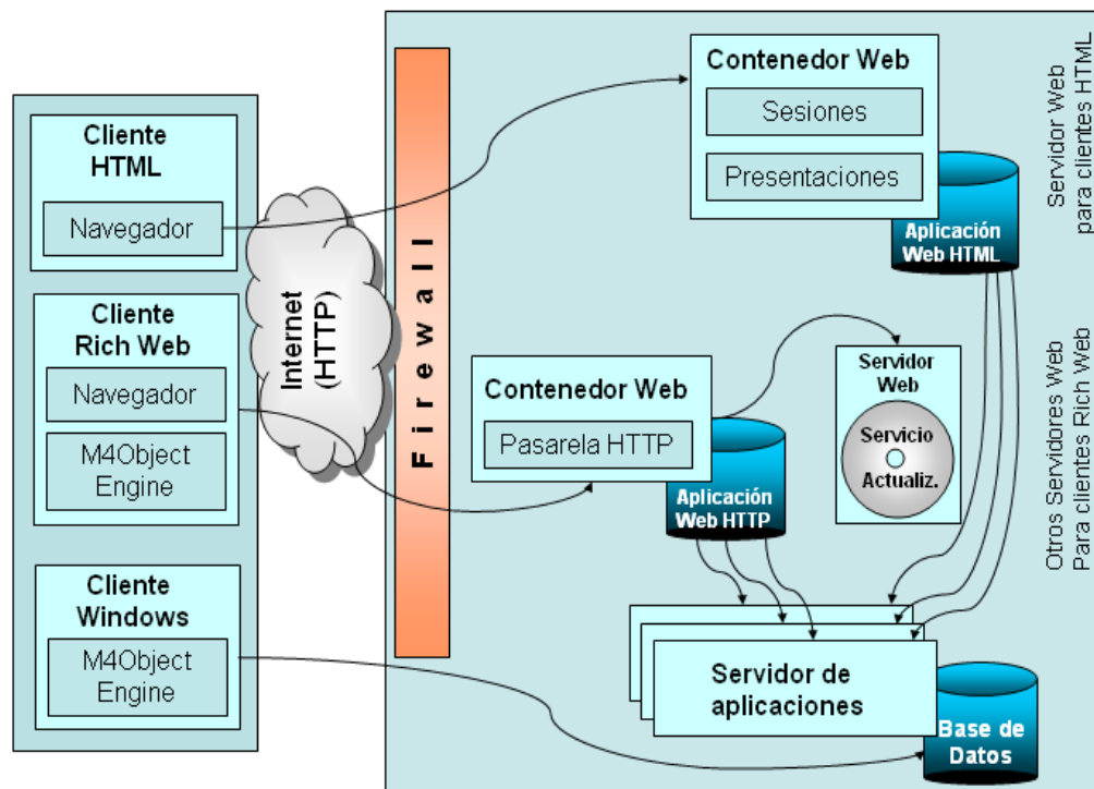
Figura 1. Arquitectura de 3 capas de Cegid con Web
