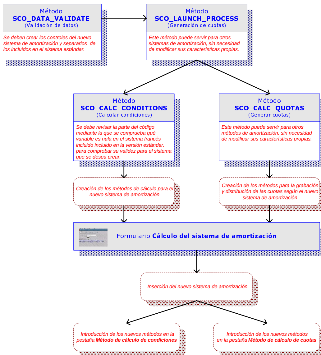
Figura 1. Esquema de las operaciones necesarias para crear un nuevo sistema de amortización
