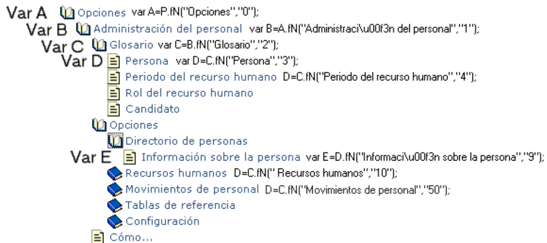
Figura 7. Árbol de ayuda en línea con sus dependencias establecidas en toc.js
