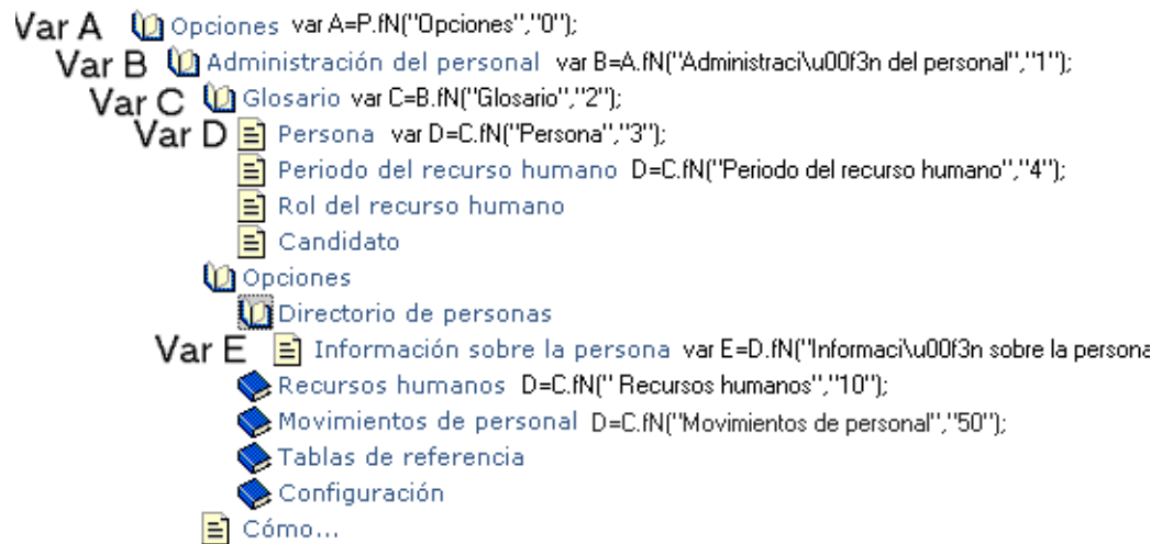
Figura 22. Árbol de ayuda en línea con sus dependencias establecidas en toc.js
