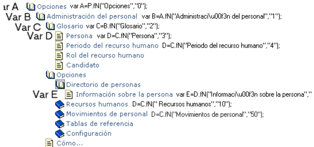
Figura 20. Árbol de ayuda en línea con sus dependencias establecidas en toc.js
