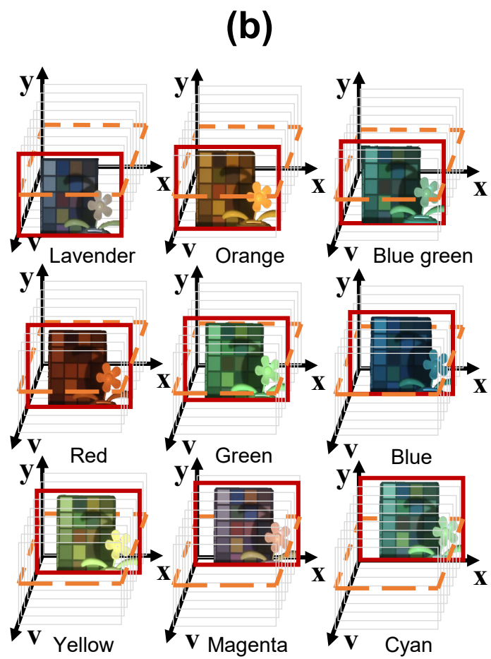
Sparse Slices
