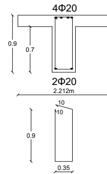
ΤΟΜΗ Α-Α
