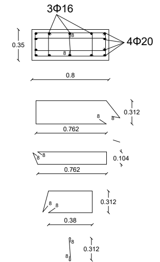
ΤΟΜΗ Δ-Δ & Ε-Ε
