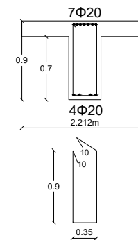
ΤΟΜΗ Γ-Γ
