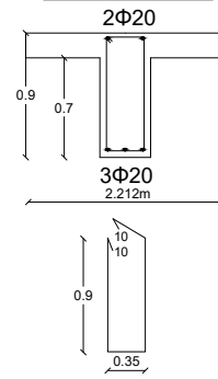
ΤΟΜΗ Β-Β
