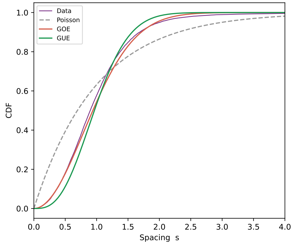
(d) Cumulative — Herm L
