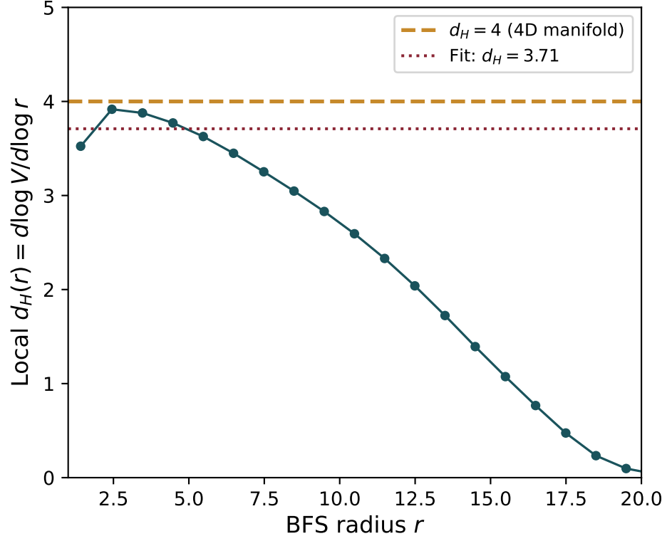
Local Hausdorff Dimension
