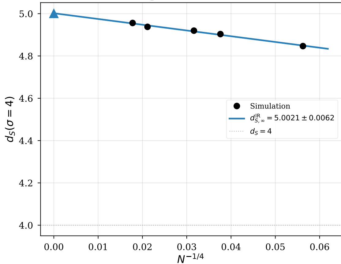
IR Spectral Dimension
