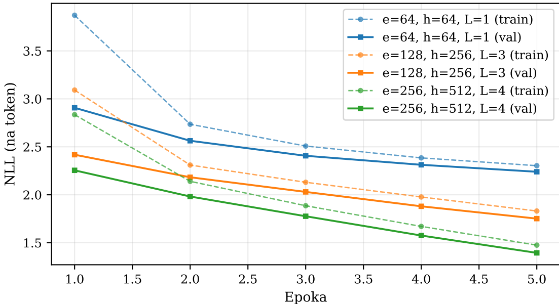
Wpływ pojemności modelu na uczenie
