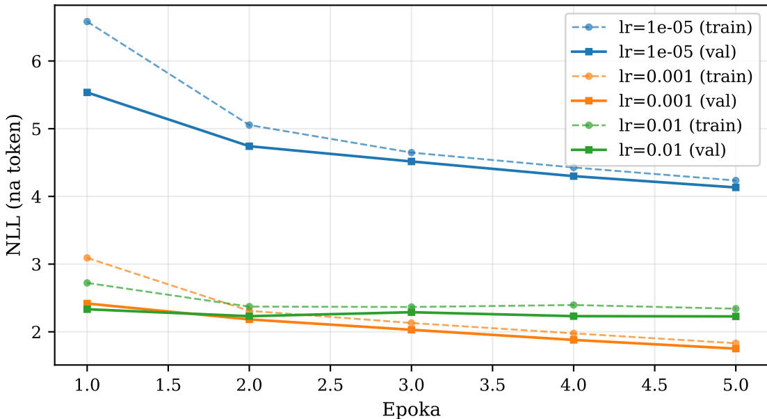
Wpływ learning rate na uczenie
