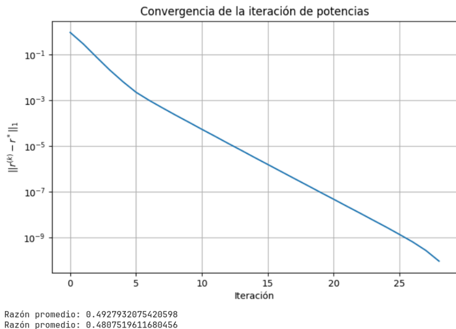
Figura 2: Convergencia de la iteración de potencias, el error decae geoméricamente.
