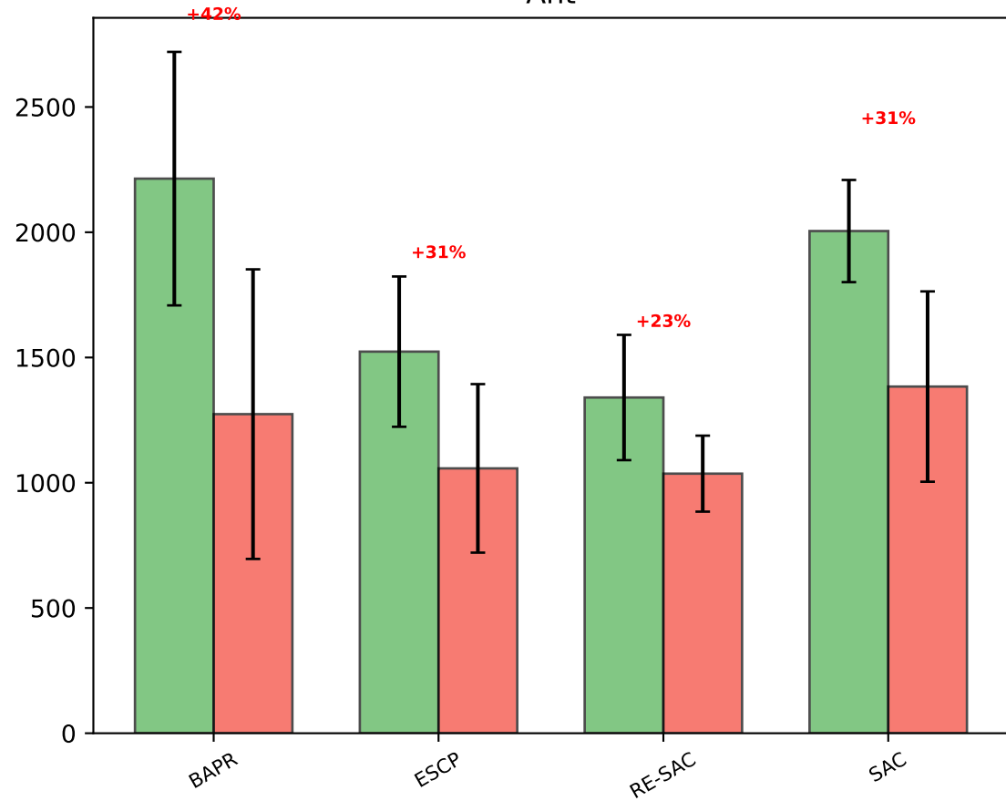
Ant
