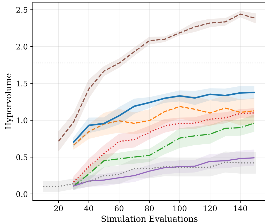
RZDT1 (convex, sqrt-noise)
