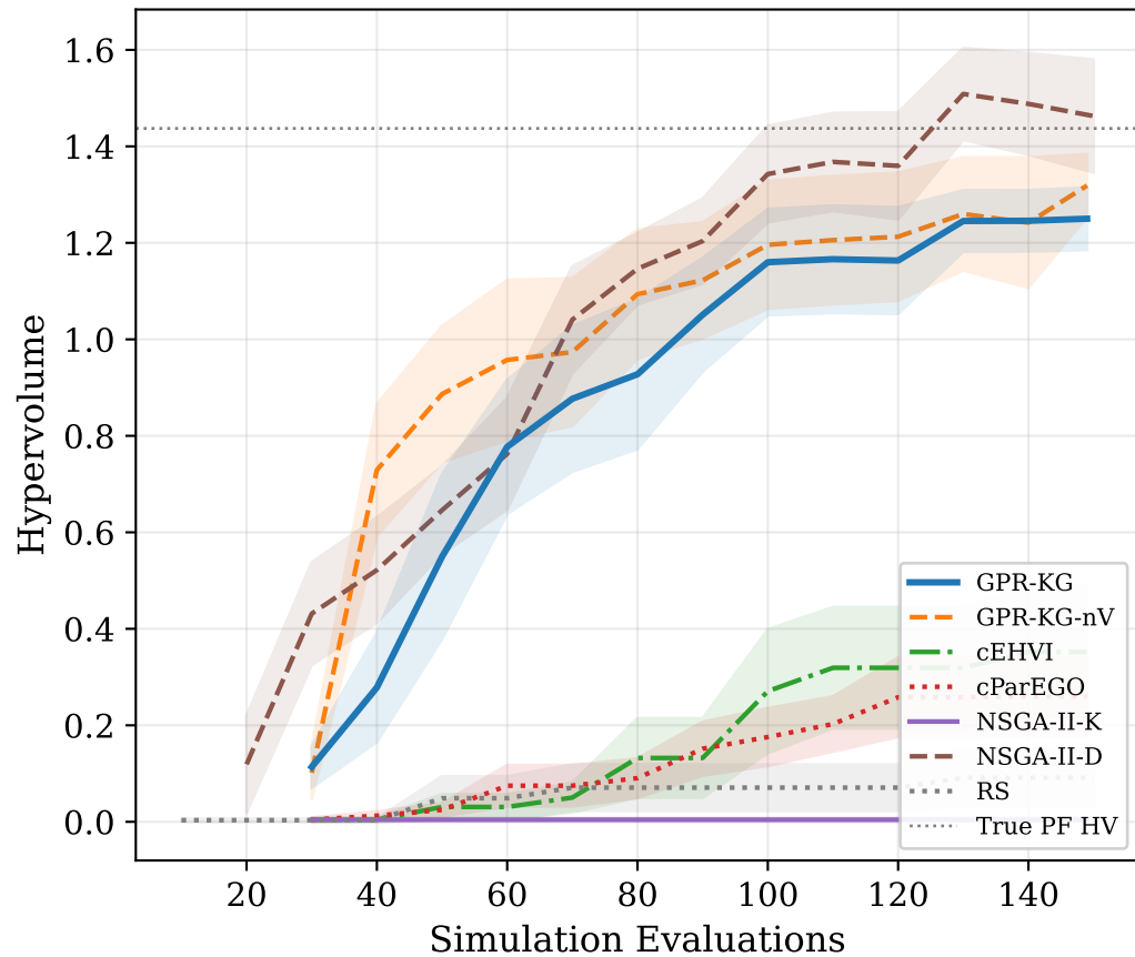
RZDT2 (concave, bell-noise)
