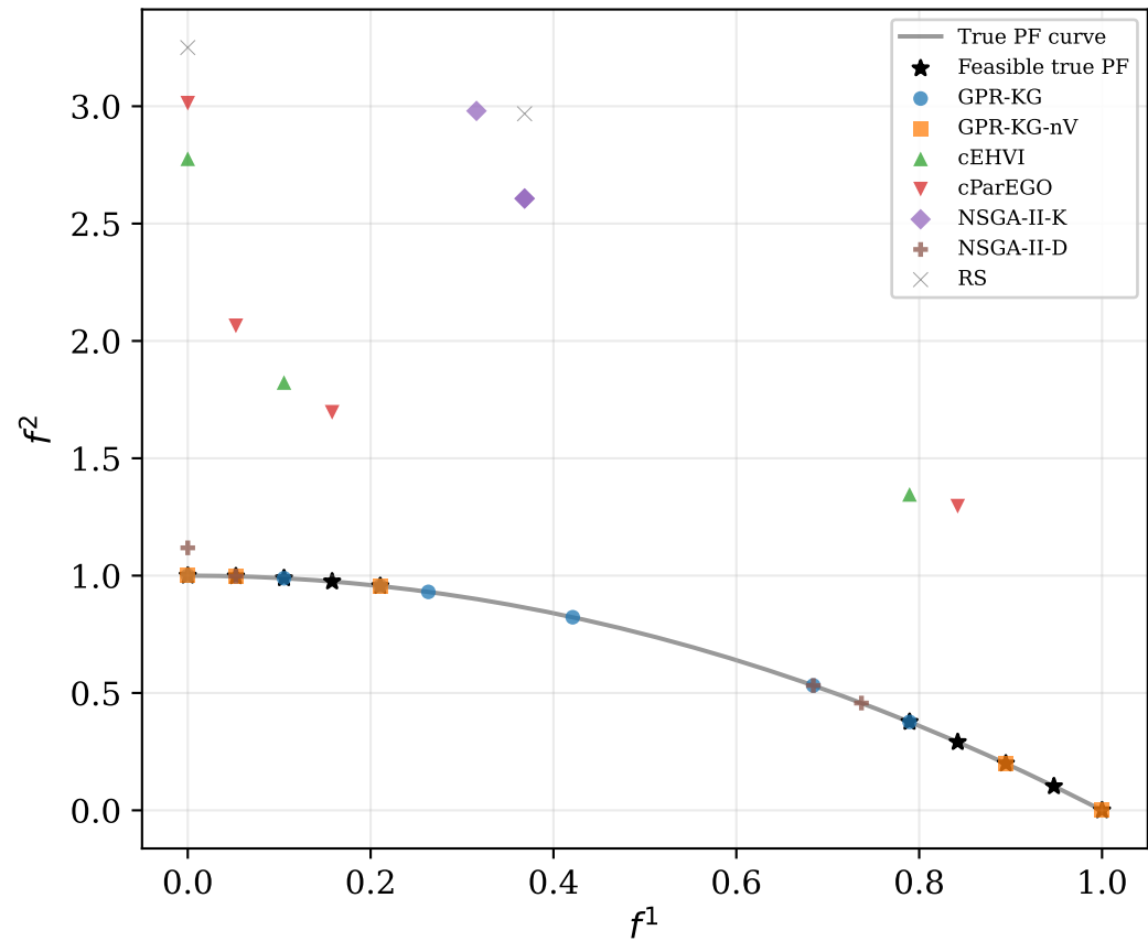
RZDT2 (concave, bell-noise)
