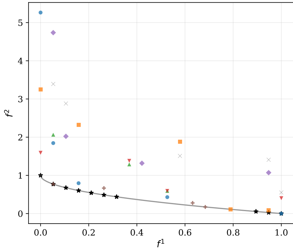
RZDT1 (convex, sqrt-noise)
