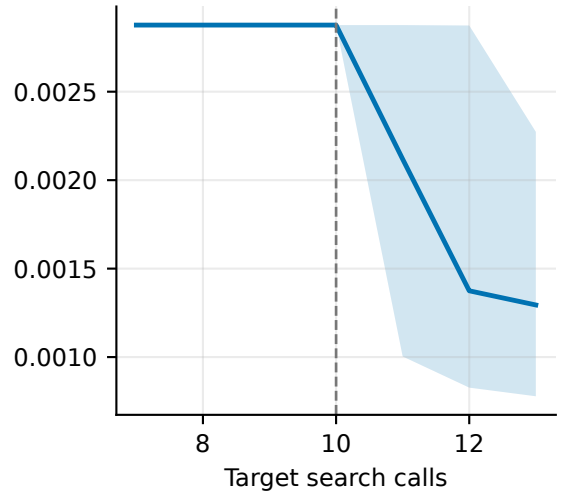
Queue
