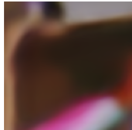
LTE 27.6384 dB
