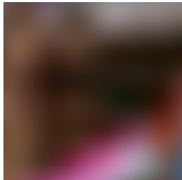
Bicubic 24.6671 dB
