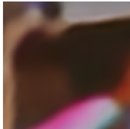
LIIF 27.5249 dB
