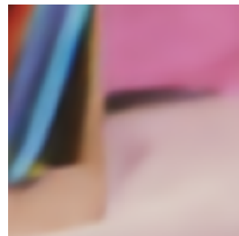
LIIF 29.4028 dB
