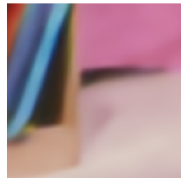
SC-INR 29.5549 dB
