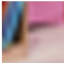
Bicubic 24.8304 dB
