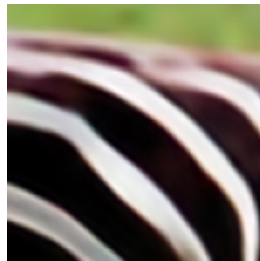
SC-INR+PhiZ 21.2201 dB
