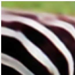
LIIF 21.1164 dB
